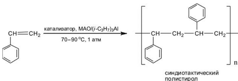
Рис. 3.50. Синтез синдиотактического полистирола
