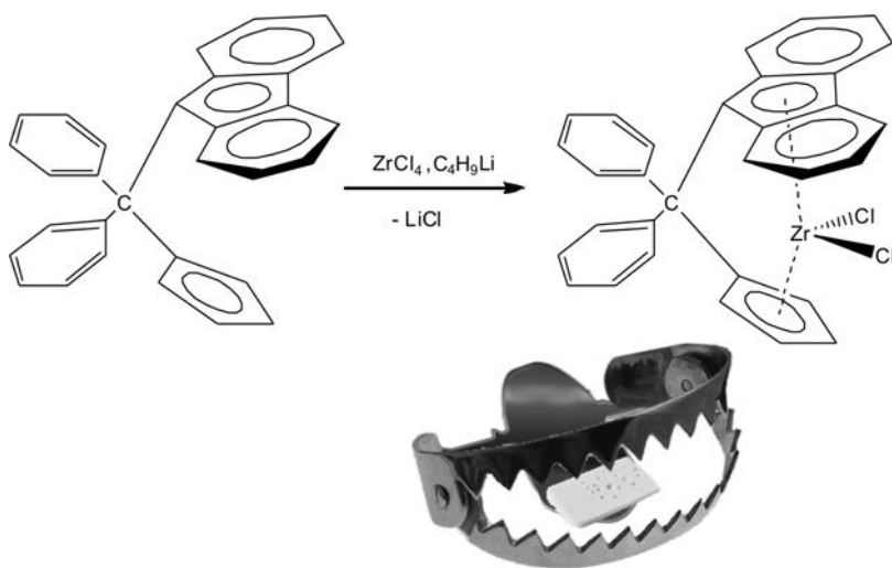
Рис. 3.47. КАТАЛИЗАТОР СИНДИОТАКТИЧЕСКОЙ ПОЛИМЕРИЗАЦИИ ПРОПИЛЕНА
