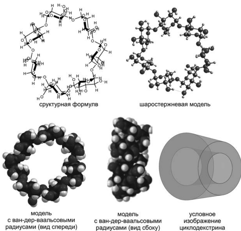
Рис. 1.46. СТРОЕНИЕ ЦИКЛОДЕКСТРИНА
