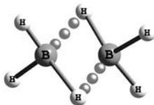
Бороводороды
