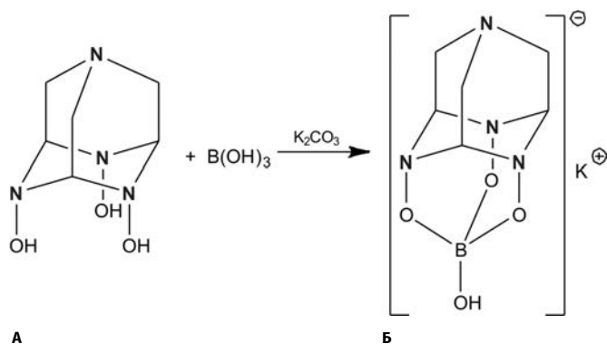
Рис. 7.50. ПОЛУЧЕНИЕ ДВУХ СПЯЯННЫХ КАРКАСОВ
