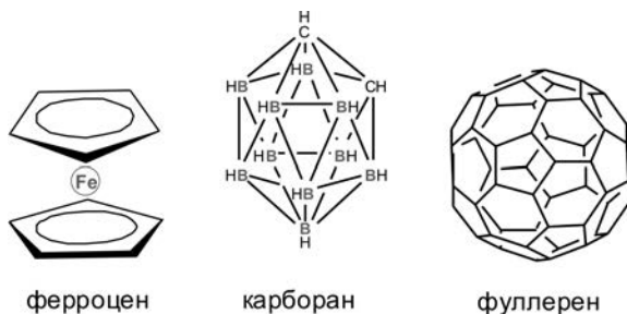
Рис. 7.37. Выдающиеся соединения XX столетия
