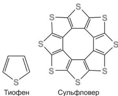
Рис. 7.38. ТИОФЕН И СУЛЬФЛОВЕР
