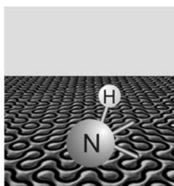
Присоединение одного атома H к атому N
