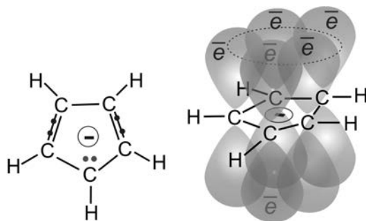
Рис. 2.20. СТРОЕНИЕ ЦИКЛОПЕНТАДИЕНИЛ-АНИОНА. ТАКАЯ ПАРА ЗАНИМАЕТ ОДНУ ОРБИТАЛЬ. НА ПРАВОМ РИСУНКЕ ЭЛЕКТРОНЫ ОБОЗНАЧЕНЫ СИМВОЛОМ e^-
