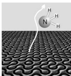
Отделение молекулы NH_3 от поверхности катализатора
