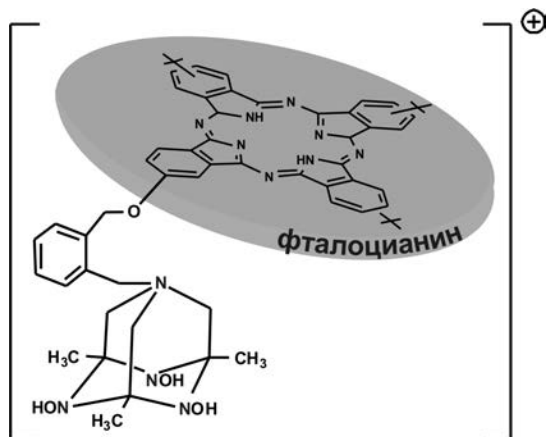
Рис. 7.53. Объединение молекул изо -уротропина и фталоцианина
