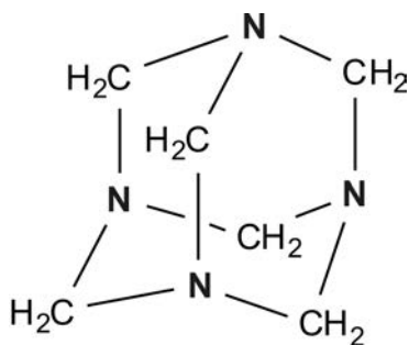
Рис. 7.39. СТРУКТУРА УРОТРОПИНА
