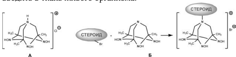
Рис. 7.52. Солянокислая соль изо -уротропина (А). Присоединение СТЕРЕИДА К ИЗО -УРОТРОПИНУ (Б)
