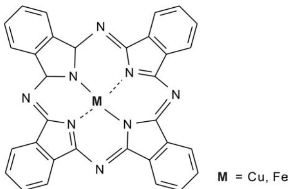
Рис. 8.28. Фталоцианиновый комплекс
