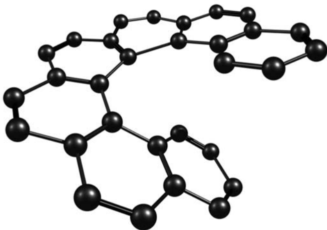
Рис. 7.13. Гелицен из бензольных циклов
