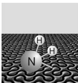
Присоединение двух атомов H к атому N
