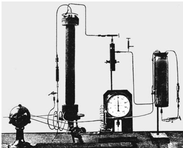
Рис. 3.12. Экспериментальная установка Ф. Габера
