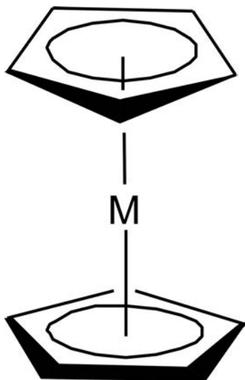
Рис. 3.44. СТРОЕНИЕ МЕТАЛЛОЦЕНА
