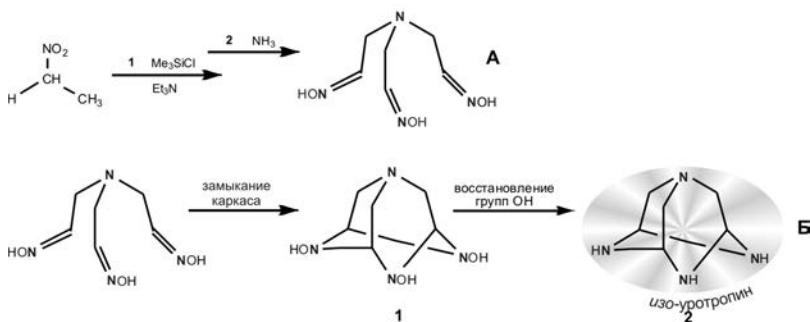
Рис. 7.46. СИНТЕЗ ИЗО-УРОТРОПИНА
