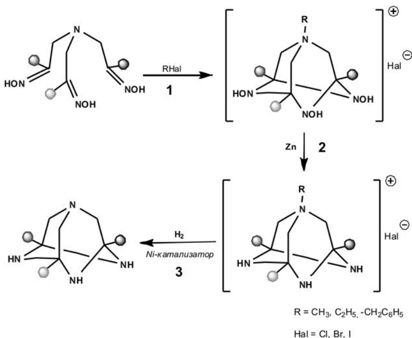
Рис. 7.47. Получение ионного соединения с тетразамещенным атомом азота в вершине каркаса (заместители в группировках \text{-CH-} показаны шариками)
