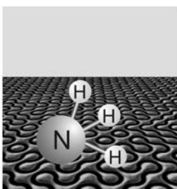
Присоединение трех атомов H к атому N
