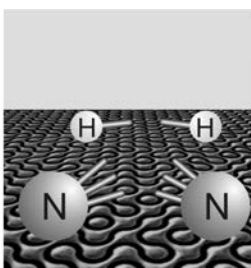
Распад двухатомных молекул на атомы (диссоциация)
