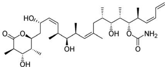
Рис. 5.46. ДИСКОДЕРМОЛИД
