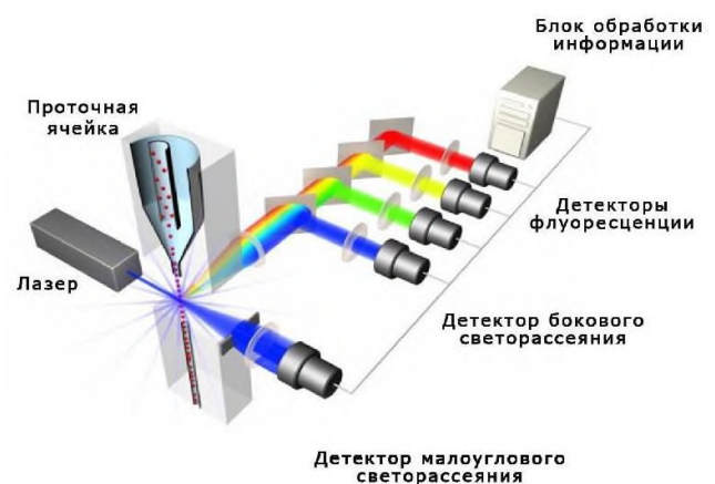
Рис.133. Принцип работы проточного цитометра.
